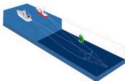
Chalut pélagique (en boeuf)
